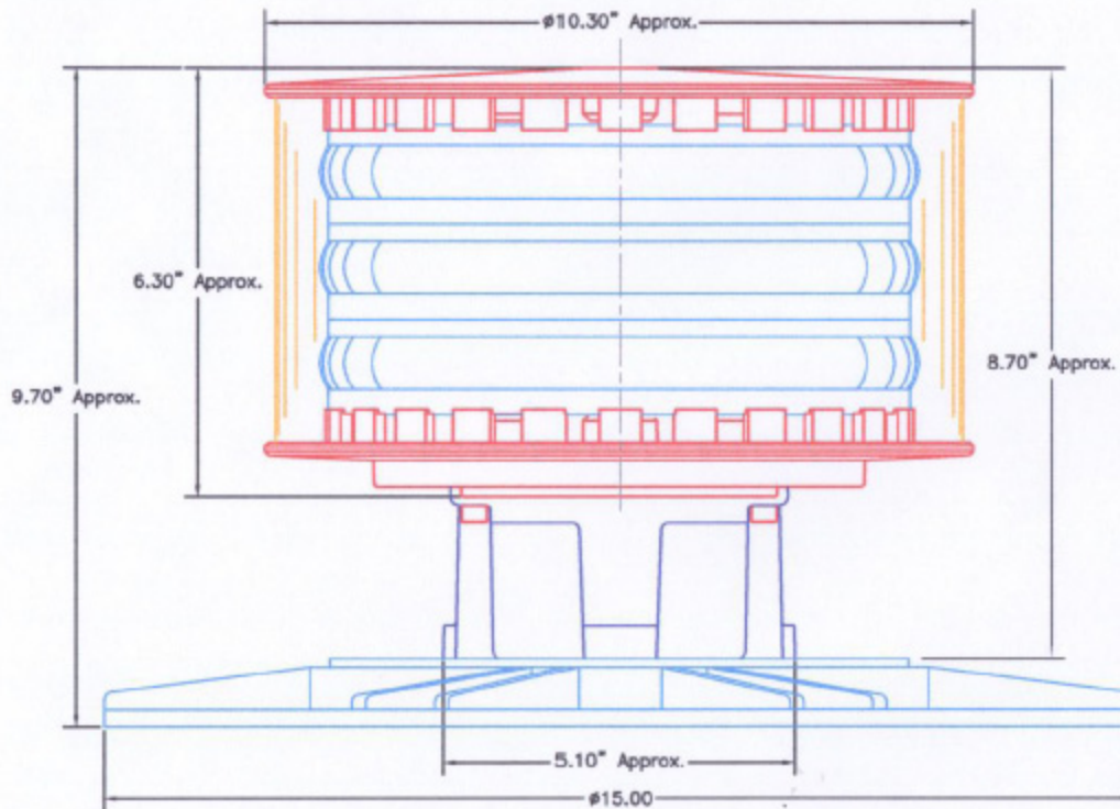
L-864LED3 BEACON LIGHT
